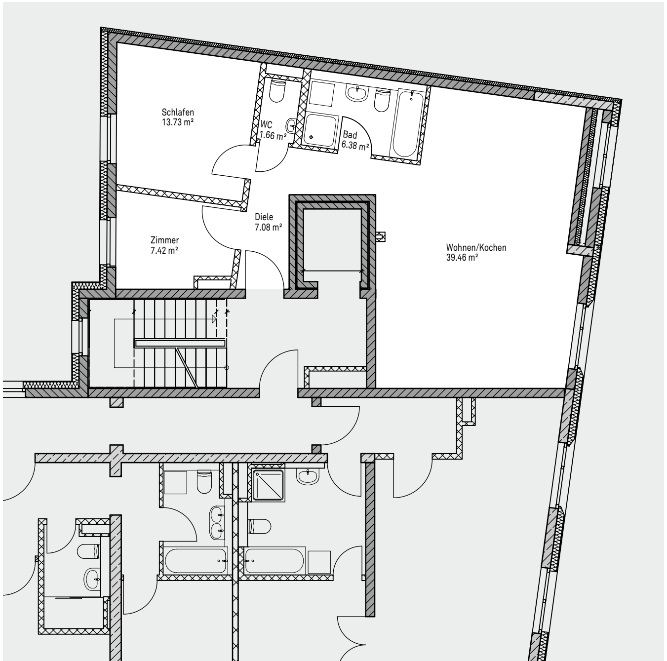
Grundriss der Wohnungen Nr. 8, 12, 16 und 20
