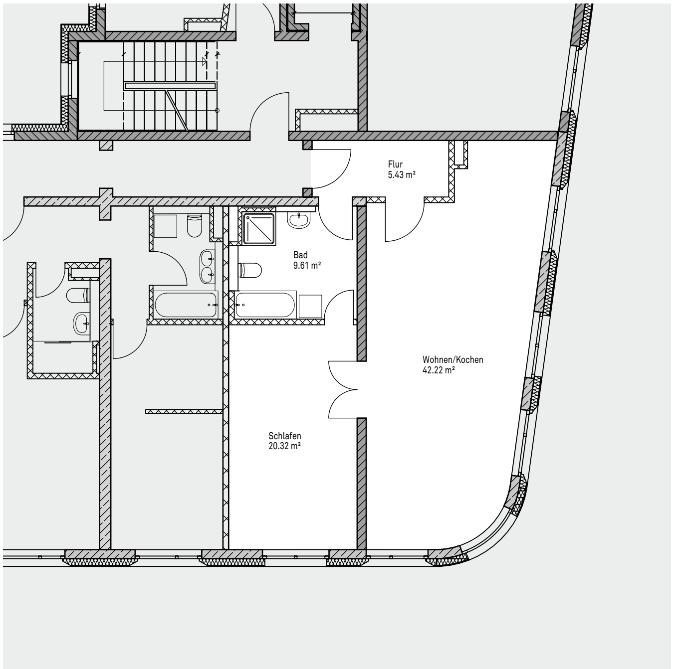
Grundriss der Wohnungen Nr. 7, 11, 15 und 19
