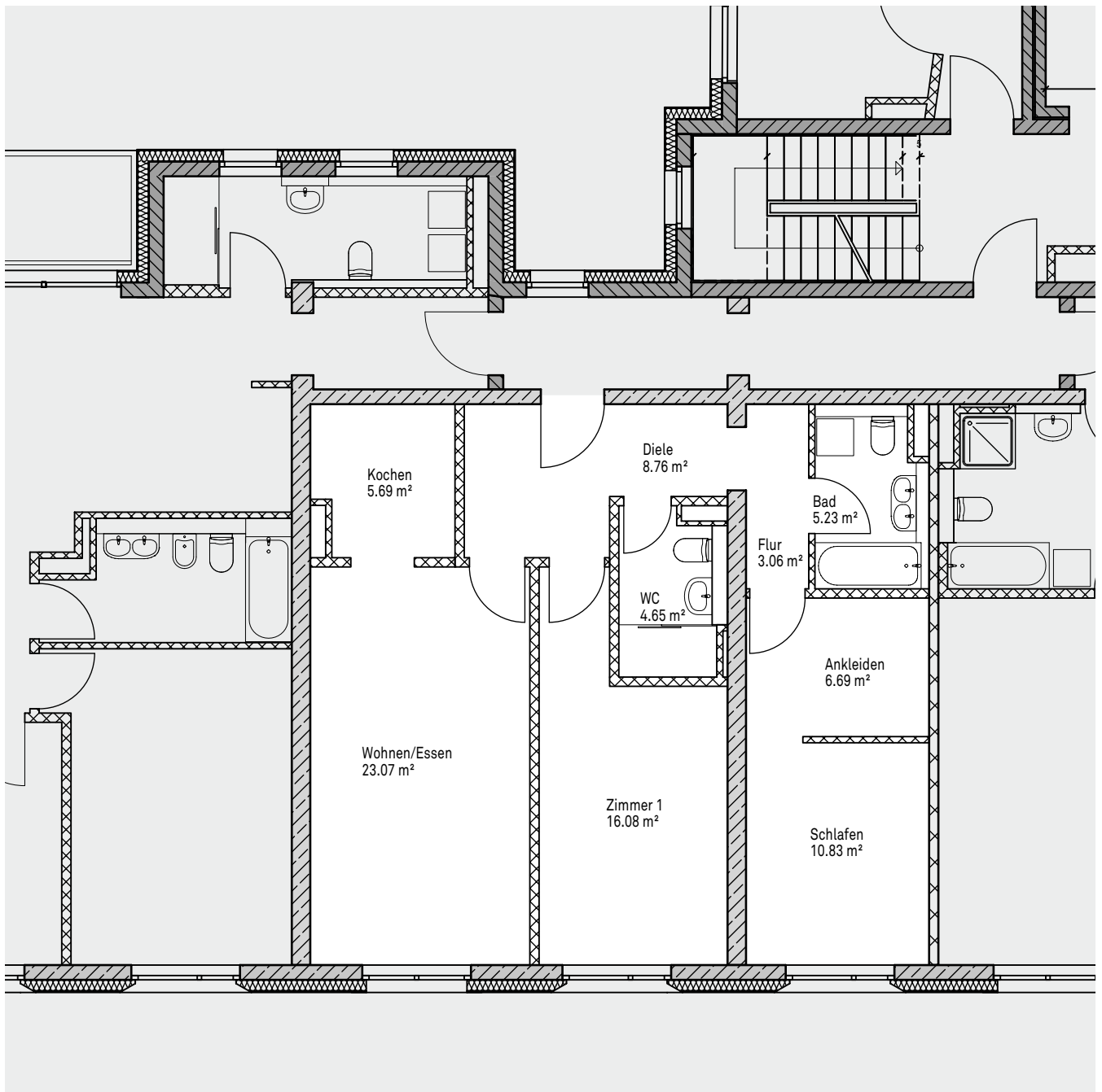
Grundriss der Wohnungen Nr. 6, 10, 14 und 18
