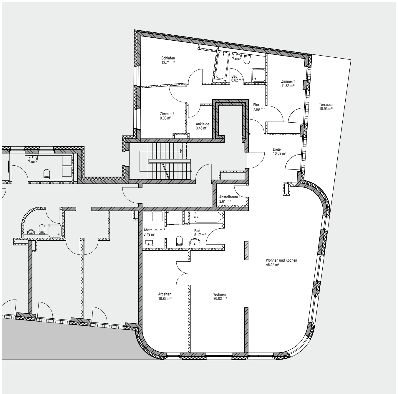
Grundriss der Wohnung Nr. 22
