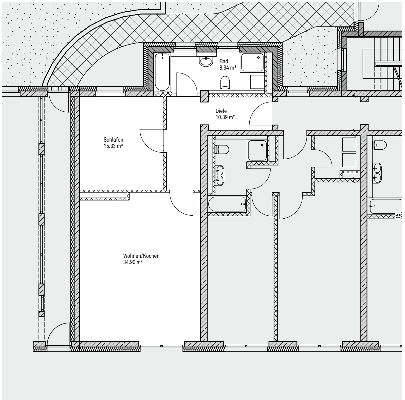
Grundriss der Wohnung Nr. 1
